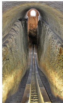
ულუგ-ბეგის ობსერვატორია
