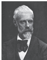
ვილჰემ ტომსენი
