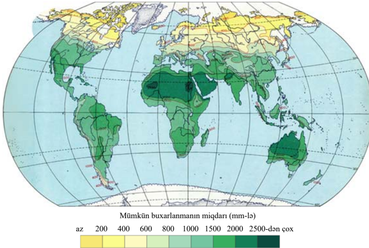
Yerdə mümkün buxarlanmanın paylanması xəritəsi
