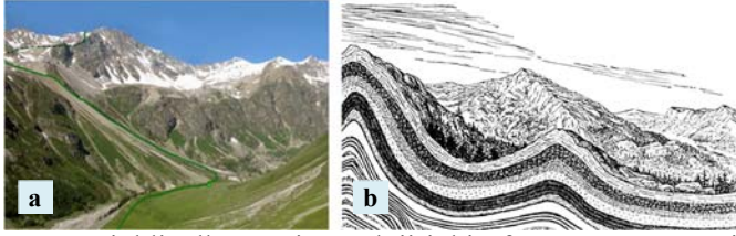
Cavan qırıxıq dağlar – geosinklinal.
