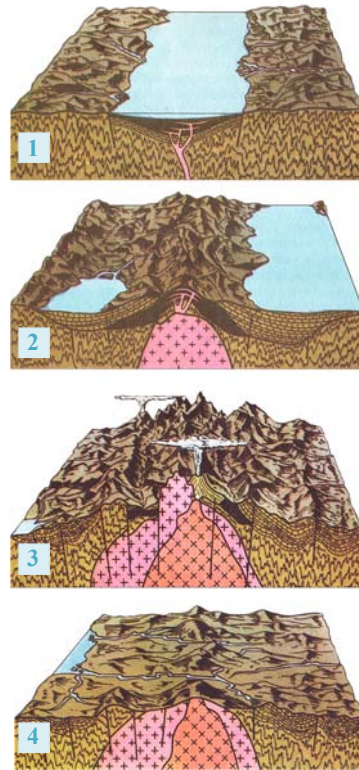
Geosinklinalın inkişaf mərhələləri
