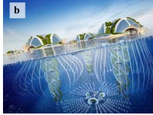
Braziliya. Okeanın dibində şəhər
