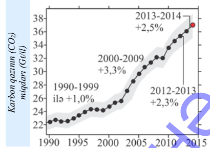
Atmosfərdə karbon qazının miqdarının dəyişməsi (1 Giqaton (Gt) = 10^9 t)
