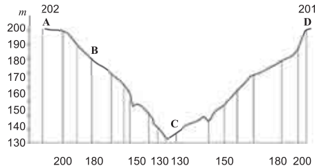
Topoqrafik xəritədə horizontlara əsasən A – D xətti üzrə ərazinin profili
