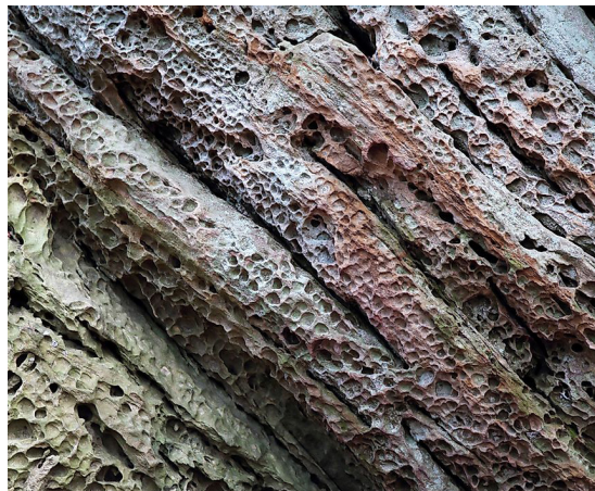
Kimyəvi aşınmanın nəticələri
