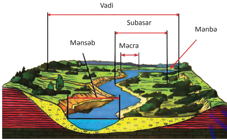
Çay yatağının elementləri
