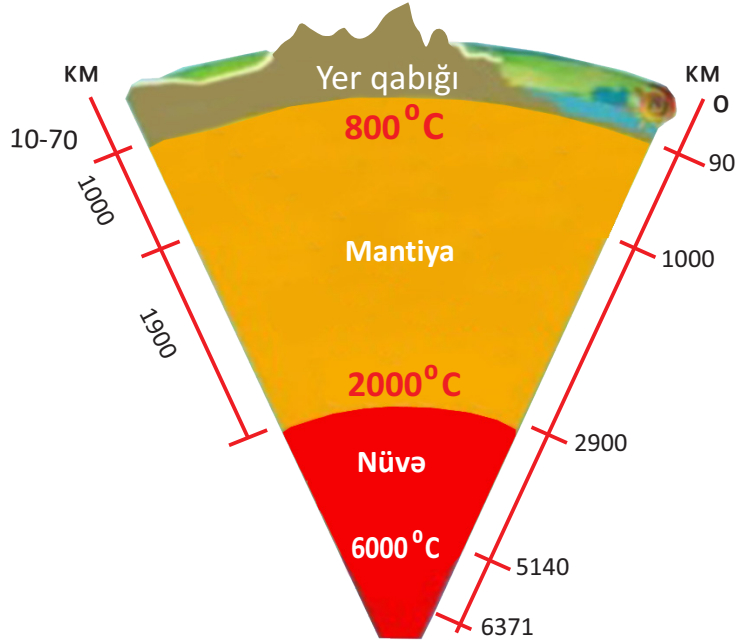
Yerın daxili quruluşu
