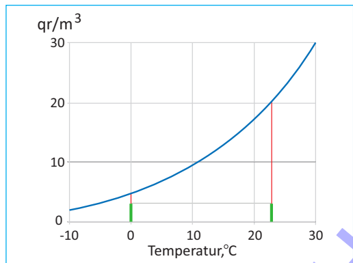
Havada olan rütubətin temperaturdan asılılığı
