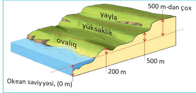
Düzənliklərin hündürlüyünə görə səviyyəsi
