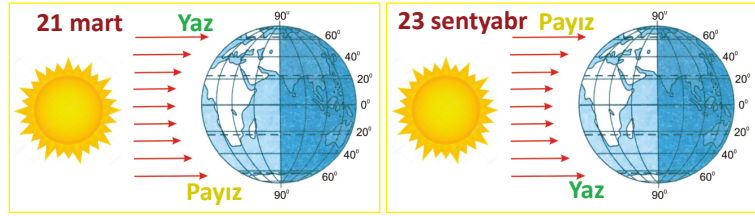
Günəşin Yer səthini bərabər qızdırması və işıqlandırması vəziyyəti
