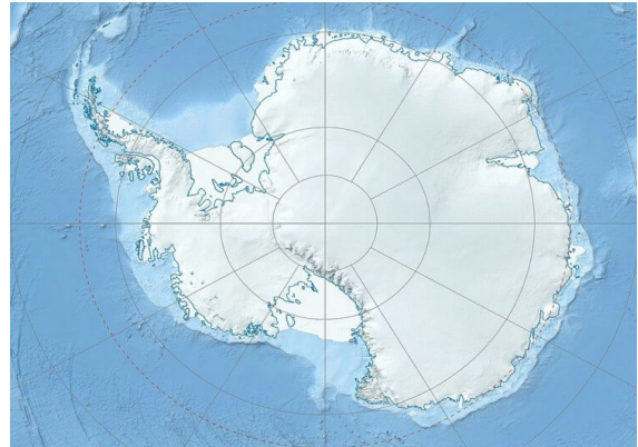
Antarktidada buz örtüyü
