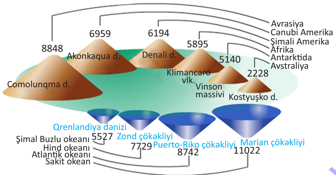
Materiklərin ən hündür zirvələri və okeanların ən dərin sahələri
