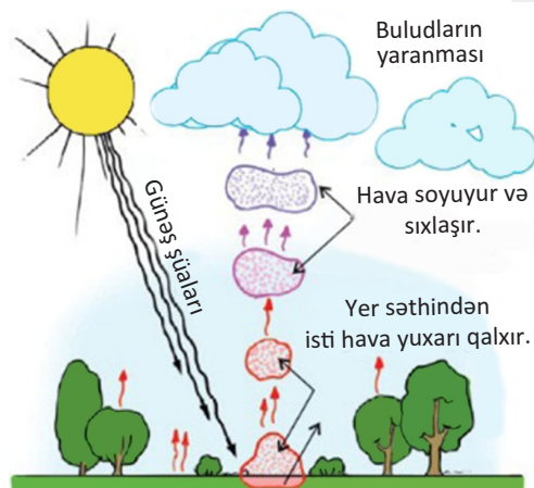
Havanın qızması və yuxarı qalxması
