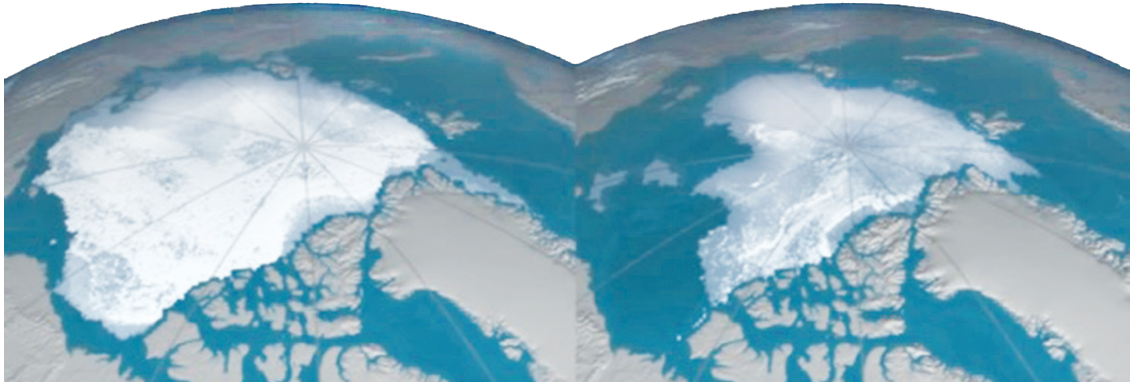
Arktikada buzların sahəsi azalır.
