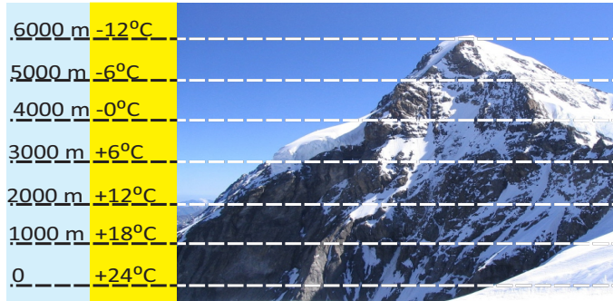
Yüksəkliyə doğru temperaturun azalması
