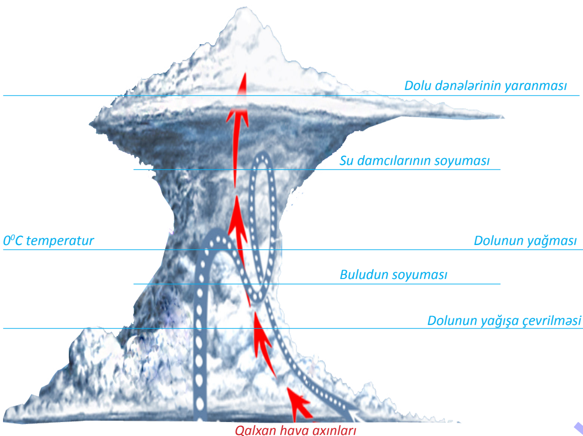
Dolunun əmələ gəlməsi
