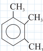
1,2,3-trimetilbenzol
