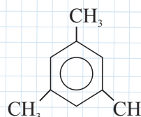
1,3,5-trimetilbenzol
