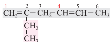
2-etilheksadien-1,4
