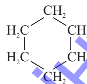
tsikloheksan
