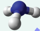
NH_3
