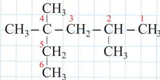
2,4,4-trimetilheksan
