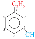
1-metil-3-etilbenzol
