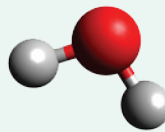
H_2O
