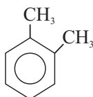
o -ksilol
