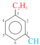
1-metil-3-etilbenzol
