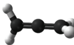
mil-kürəcik modeli
