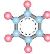
Benzol molekulunun mil-kürəcik modeli
