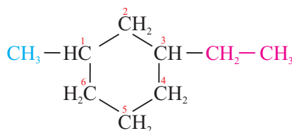
1-metil-3-etiltsikloheksan
