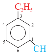
1-metil-3-etilbenzol
