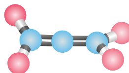
mil-kürəcik modeli
