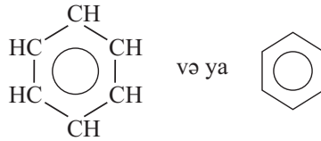
Benzol molekulunun qrafik formulu
