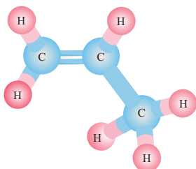
Propen molekulunun mil-kürəcik modeli
