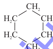
tsikloheksan
