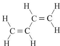
qrafik formul
