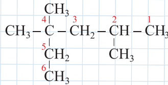
2,4,4-trimetilheksan
