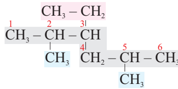
2,5-dimetil-3-etilheksan
