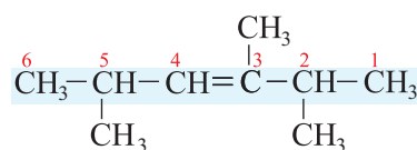
2,3,5-trimetilheksen-3
