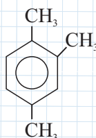
1,2,4-trimetilbenzol
