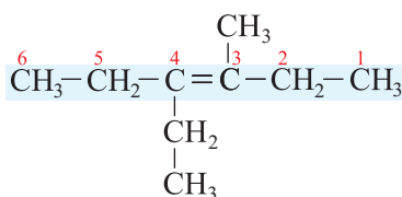
3-metil-4-etilheksen-3
