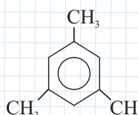
1,3,5-trimetilbenzol
