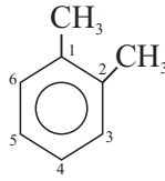
1,2-dimetilbenzol
