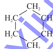
tsikloheksan
