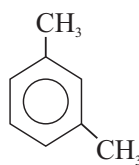
m-ksilol
