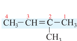
2-metilbuten-2
