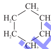
tsikloheksan
