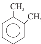
o-ksilol
