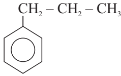
propilbenzol
