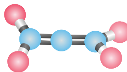
mil-kürəcik modeli
