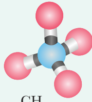
CH_4
