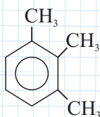
1,2,3-trimetilbenzol
