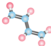
mil-kürəcik modeli
