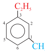
1-metil-3-etilbenzol
