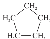
tsiklopentan
