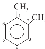
1,2-dimetilbenzol
