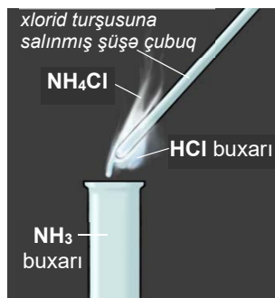
(f) "Alovsuz tüstü"
