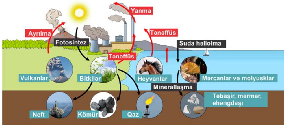
(a) Təbiətdə karbon dövrəni
