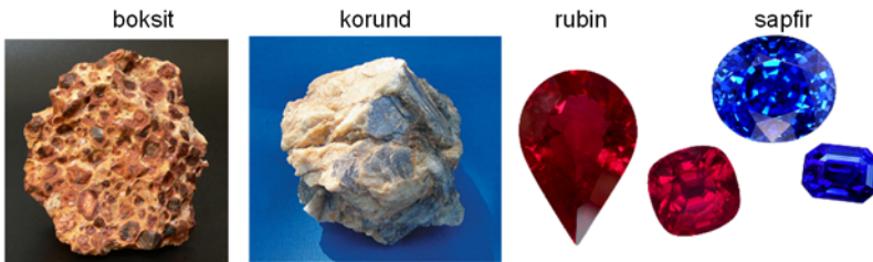
(d) Alüminium-oksidi təbii mineralları
