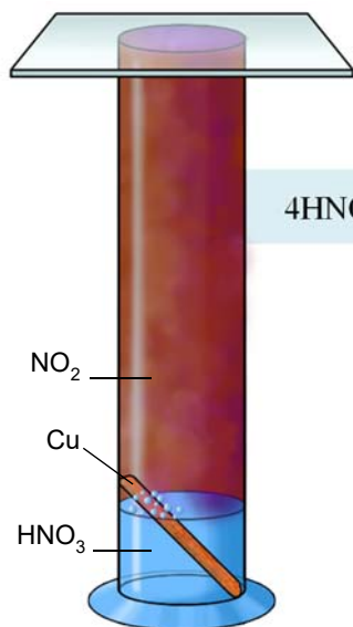
(c) Qatı nitrat turşusunun mislə qarşılıqlı təsiri
