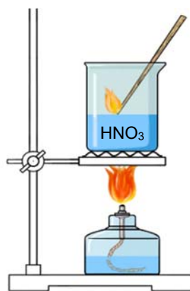
(a) Zəif közərdilmiş çubuğun qızdırılmış qatı nitrat turşusunda alışması
