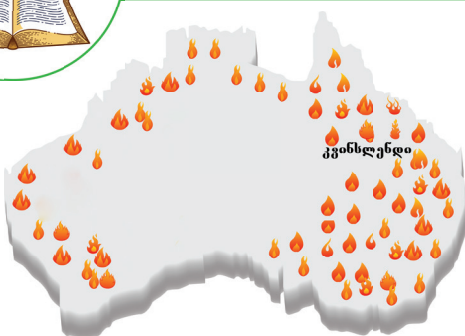
ხანძრის ზონები ავსტრალიაში 2019 წელს
