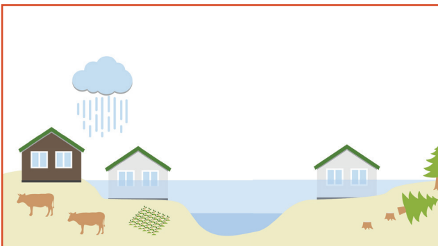
მდინარეში წყლის დონის აწევა
