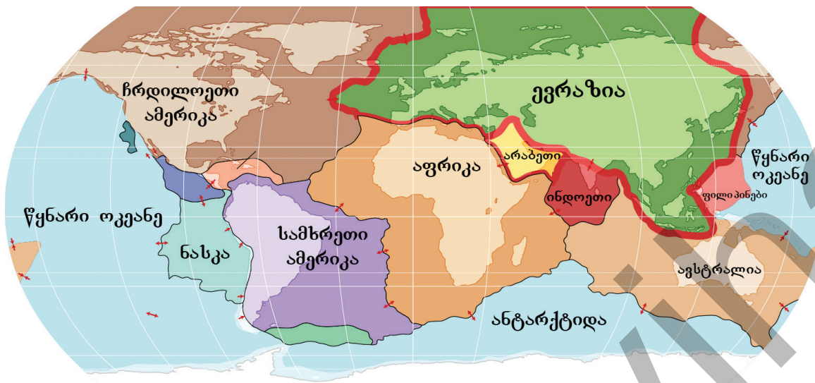
ლიტოსფეროს ფილების მოძრაობა
