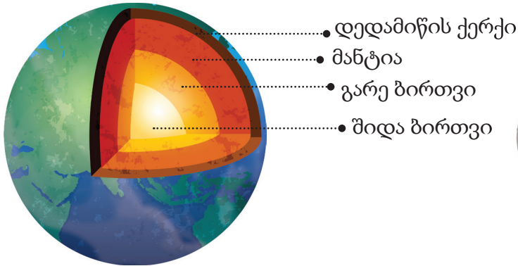
დედამიწის შიდა ფენები
