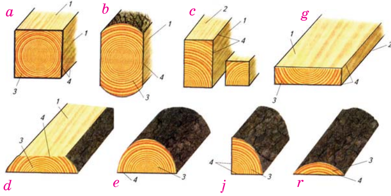
Şək. 3. Mişar materialları. a – dördhaşiyəli tir; b – ikihaşiyəli tir; c – kiçik tirlər; g – kənarları kəsilmiş taxta; d – tilləri oval taxta; e – lövhə; j – şalbanın dördə bir hissəsi; r – şalban yanı; 1 – təbəqə (lay); 2 – kənar; 3 – en kəsik (təpə); 4 – til
