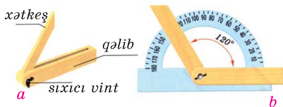
Şək. 10. Günyə və transportirlə nişanlama üsulları a —taxta günyə; b – günyənin transportir boyunca yerləşdirilməsi
