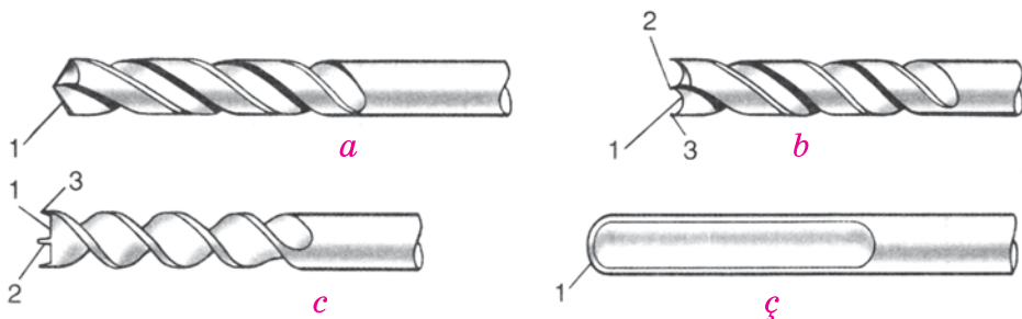
Şəkl. 2. Burğular: a – spiralvarı; b – mərkəzvarı, c – şnekvarı; ç – qaşıqvarı (1 – kəsən kənarı; 2 – mərkəz; 3 – kəsici)
