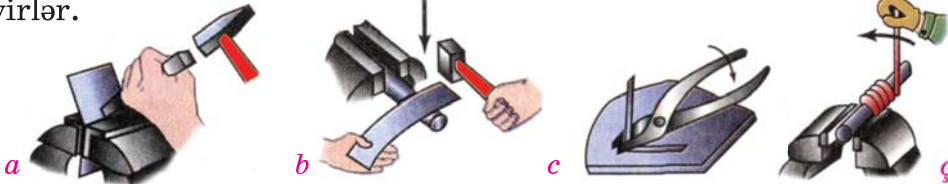
Şəkl. 2. Pəstahın əyilməsi: a – məngənədə; b – sığanaqda; c – yumruağız kəlbətinlə; ç – əymə tərtibatında
