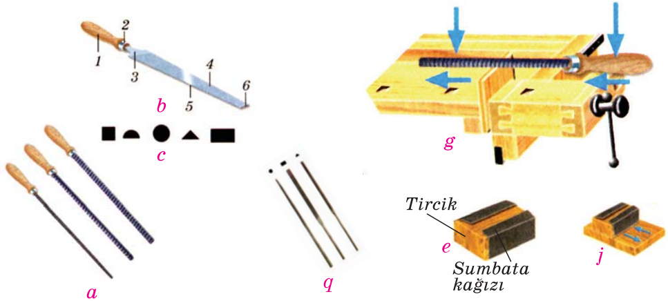
Şək. 6. Oduncaqdan olan detalların təmizlənməsi üçün alət və tərtibatlar* : a – törpülər; b – yeyənin əsas hissələri: 1 – dəstək; 2 – üzük; 3 – daban; 4 – tircik; 5 – çərtmə; 6 – uc hissəsi; c – yeyələrin profilləri (kəsikləri); q – suvandlar; g – törpü ilə təmizləmə; e – tircikli sumbata kağızı; j – sumbata kağızı ilə işləmə üsulları
