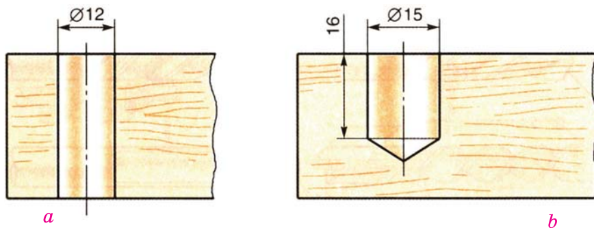
Şəkl. 1. Deşiklər: a – iki tərəfi açıq; b – bir tərəfi açıq
