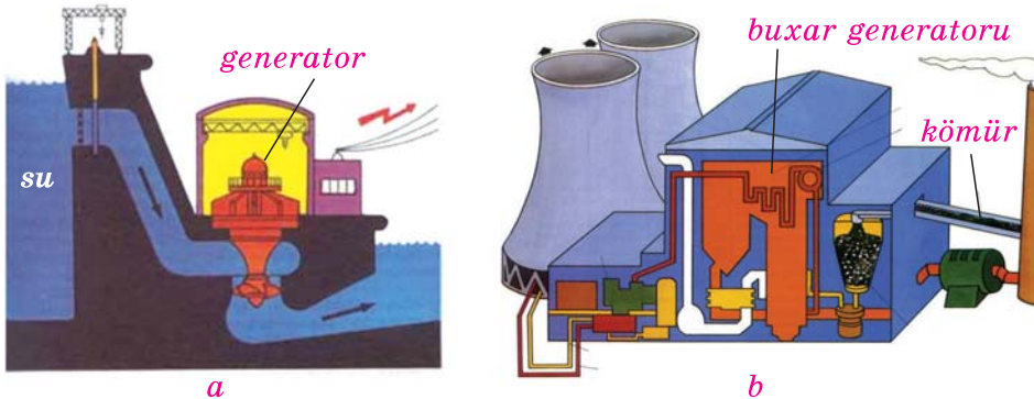
Şək. 2. Elektrik enerjisinin alınması
