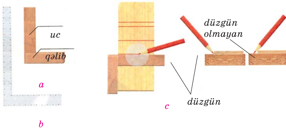
Şək. 7. Düzgün bucaqlıqları:
