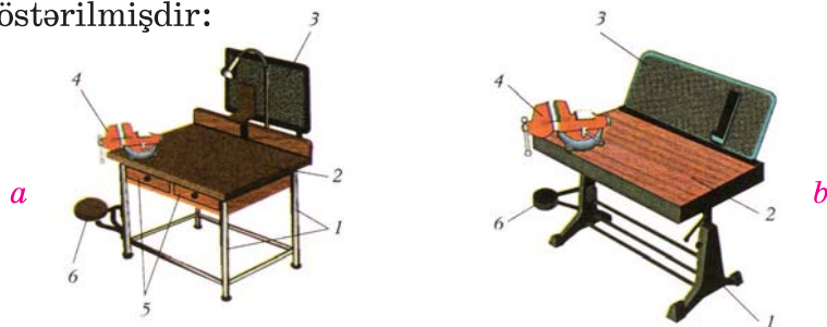
Şək. 1. Verstaklar: a – çilingər verstakı; b – kombinə edilmiş verstak: 1 – metal karkas; 2 – stolüstü (qapaq); 3 – qoruyucu tor (ekran); 4 – mənəgə; 5 – alətlər üçün yexiklər; 6 – oturmaq
