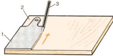
Şək. 1. Ülgü ilə nişanlama
