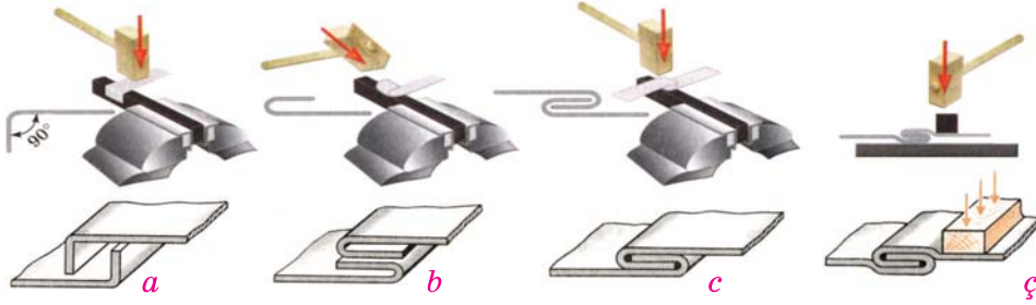
Şək. 1. Qatlama birləşdirilməsinin alınma ardıcılığı
