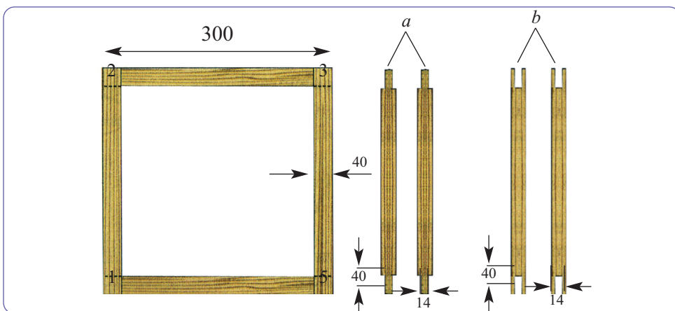
Şəkil 1. Nəfəslük üçün torlu çərçivə: a – zivana tirciklər; b – yarıqlı tirciklər
