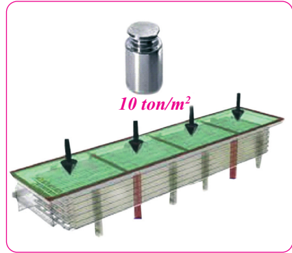
Şəkil 4. Mişar materiallarının sıxılmış vəziyyətdə qurudulması
