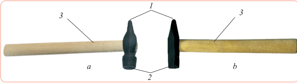
Şəkil 3. Çilingər çəkiçləri: a – dairəvidöyəcli; b – kvadratdöyəcli: 1 – burun; 2 – döyəc; 3 – dəstək
