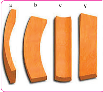
Şəkil 3. Taxtanın əyilmə növləri: a, b – uzununa; c – eninə; ç – vintvari
