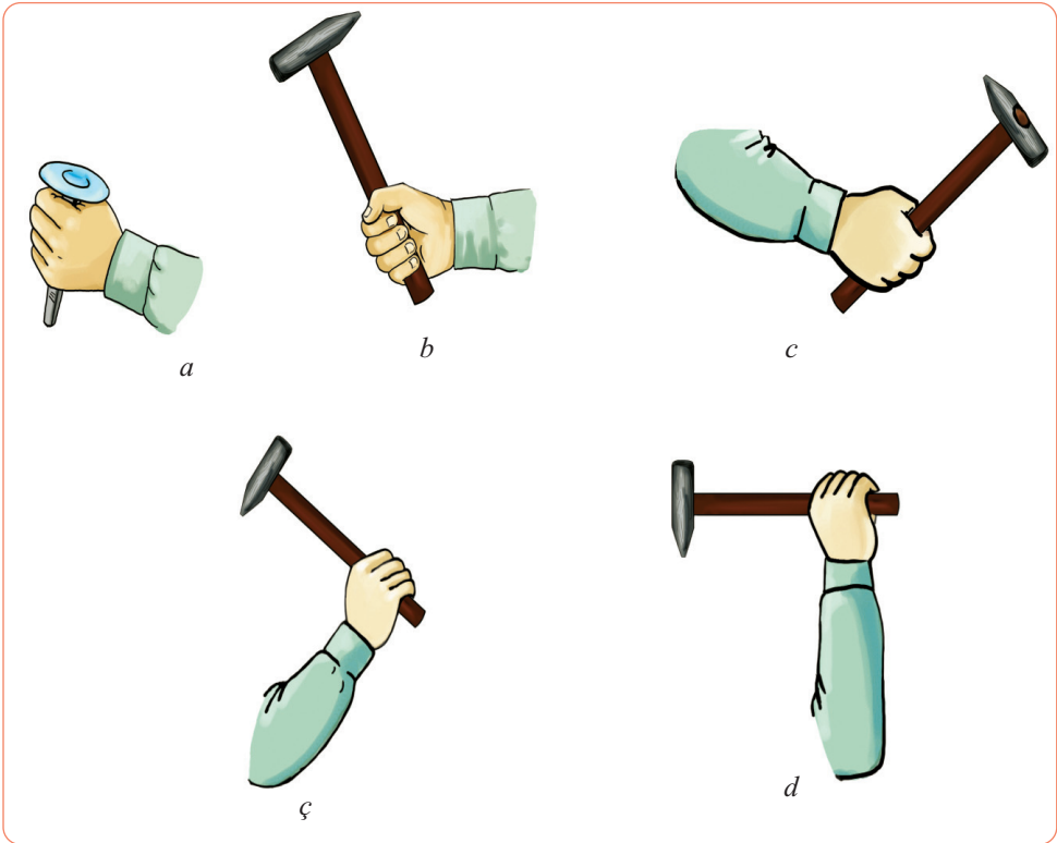
Şəkil 6. a – qələmin tutulması; b – çəkicin tutulması; c – bilək zərbəsi; ç – dirsək zərbəsi; d – çiyin zərbəsi
